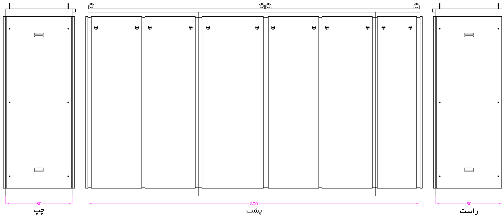
شکل ۲: نمای خارجی تابلوهای توزیع عمومی داخلی ۲۵۰۰ آمپری - پشت و چپ و راست
