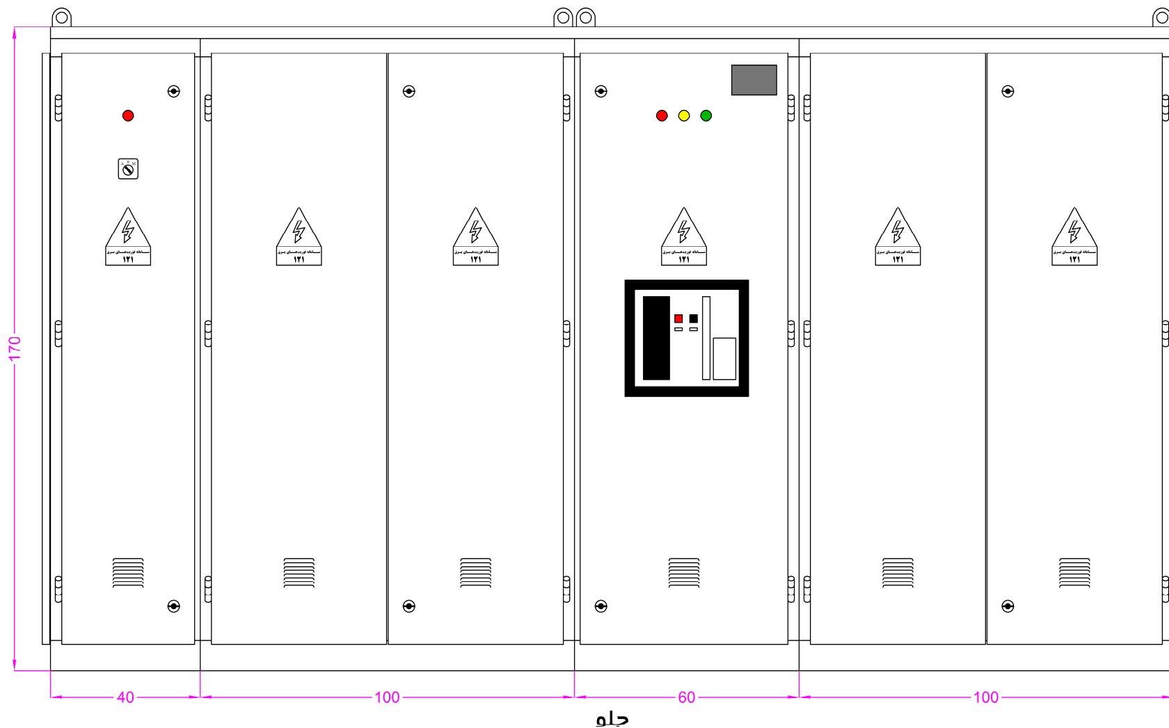
شکل ۱: نمای خارجی تابلوهای توزیع عمومی داخلی ۲۵۰۰ آمپری - جلو
