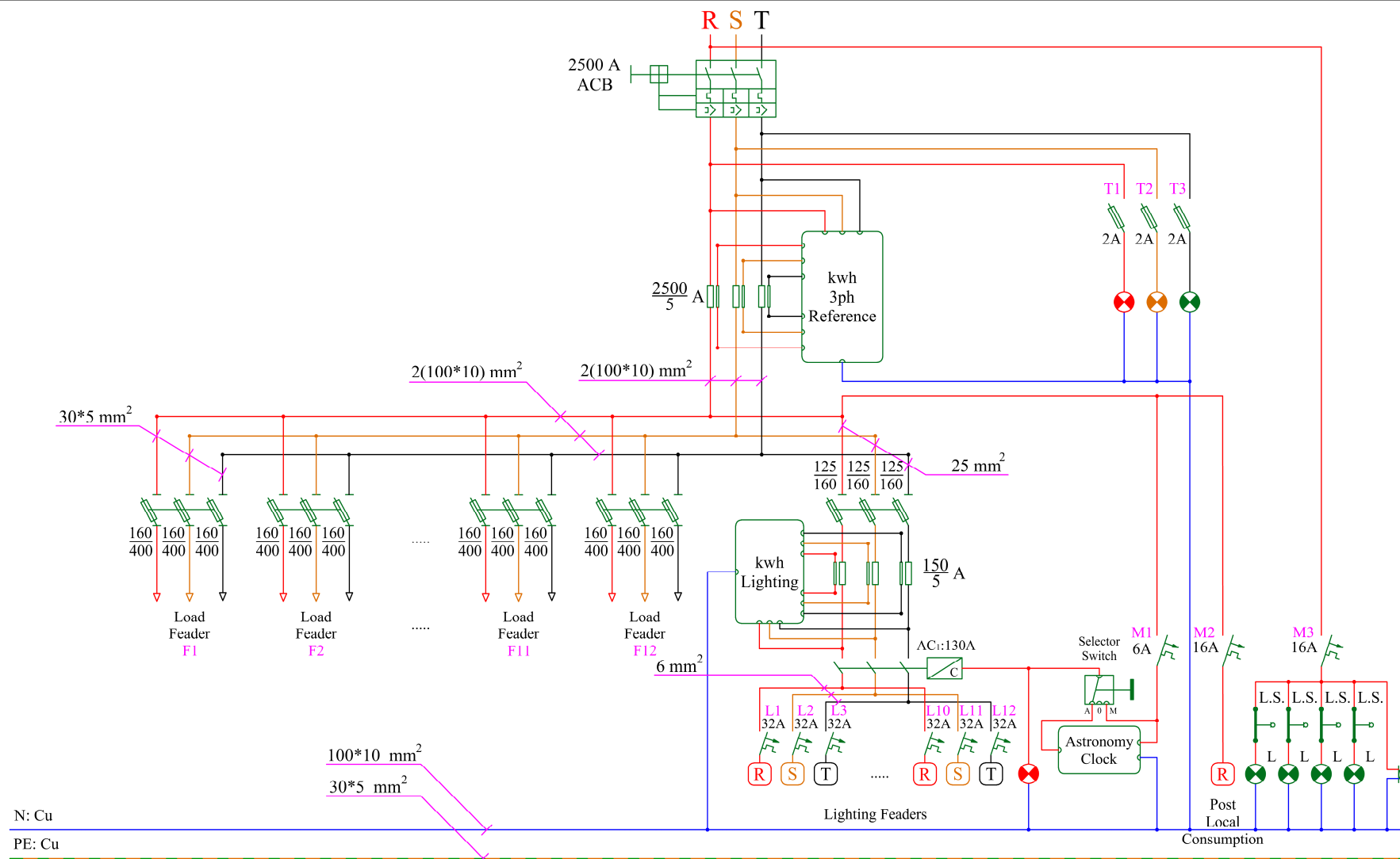
شکل ۵: دیاگرام تک خطی تابلوهای توزیع عمومی داخلی ۲۵۰۰ آمپری
